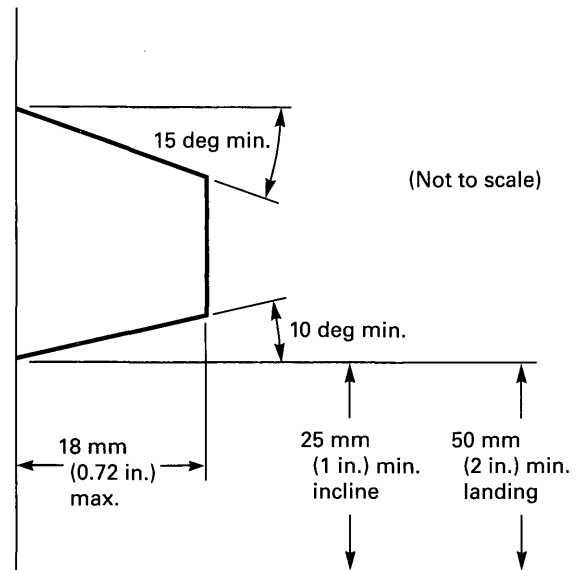
Fig. 6.1.3.3.10 Dimensions
