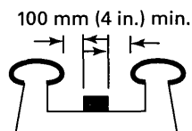
Fig. I-6 Antislid Device (6.1.3.3.10)
